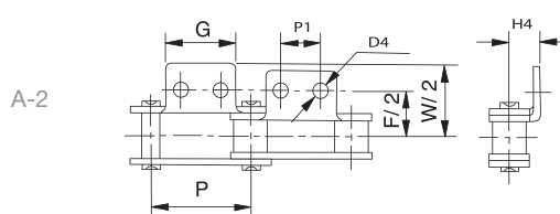
Aleta 90° 2 taladros 1 lado Attachment 90° 2 holes 1 side Équerre 90° 2 trous 1 côté
