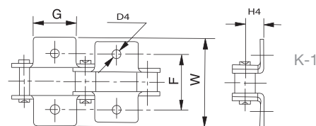
Aleta 90° 1 taladro 2 lados Attachment 90° 1 hole 2 sides Équerre 90° 1 trou 2 côtés
