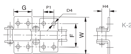
Aleta 90° 2 taladros 2 lados Attachment 90° 2 holes 2 sides Équerre 90° 2 trous 2 côtés
